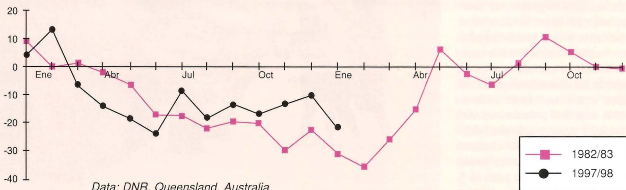
1997/98 Y 1982/83 COMPARACIÓN DE LAS VARIACIONES DEL NIVEL DEL MAR
